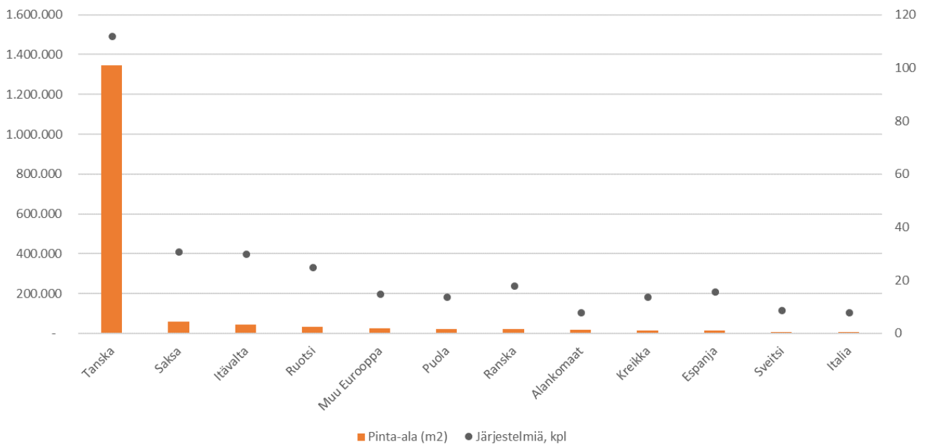
Kuva 2: Aurinkokaukolämpö ja -jäähdytys - keräinpinta-ala ja määrä järjestelmiä 2016
