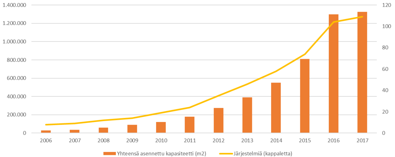
Kuva 3: Asennettu aurinkokeräinkapasiteetti kaukolämpöjärjestelmissä Tanskassa ja määrä järjestelmiä
