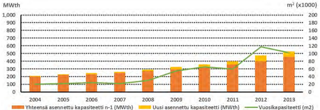
Kuva 5: Tanskan aurinkolämpömarkkinat yhteensä ja uusi asennettu kapasiteetti
