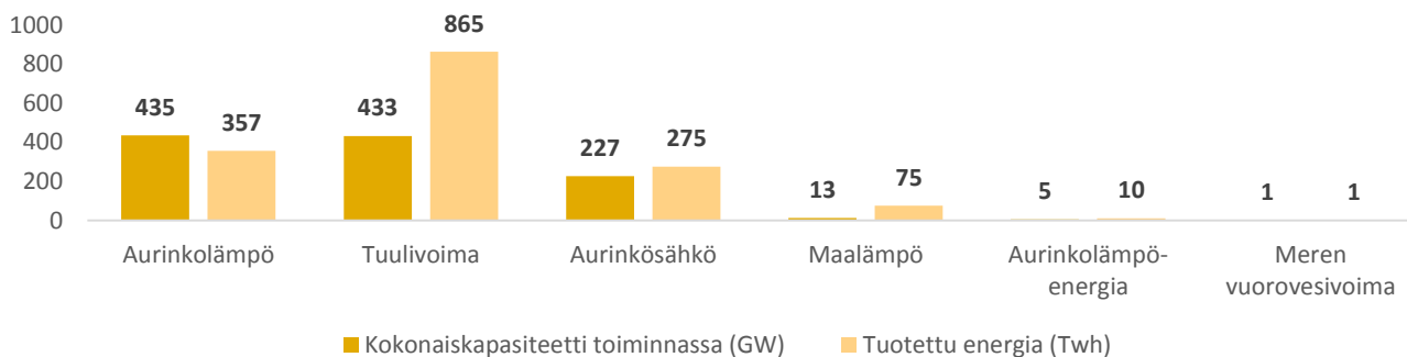
Kuva 1: Tuotannon kokonaiskapasiteetti ja tuotettu energia maailmanlaajuisesti vuonna 2015.
